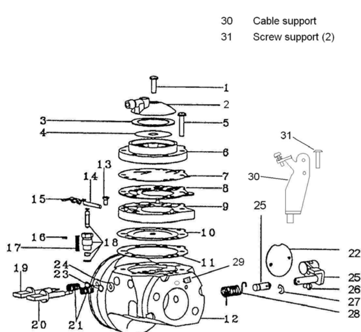
DESCRIPTION DU CARBURATEUR ET ESQUISSE DES PIÈCES
