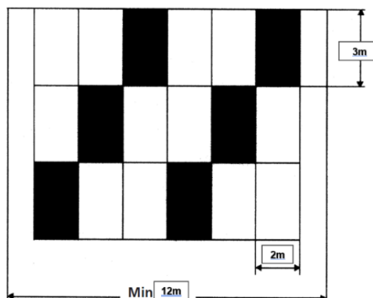
Ruudukon mitat
